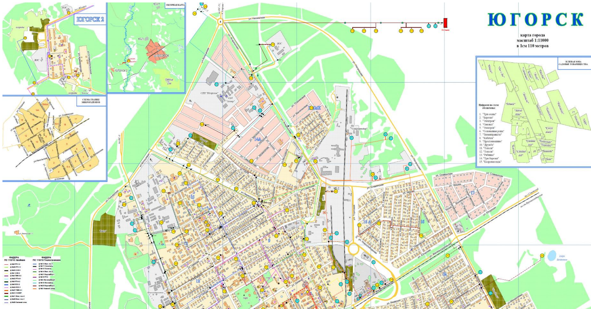
Рисунок 3.4. Карта схема сетей электроснабжения муниципального образования город Югорск (часть 1)
