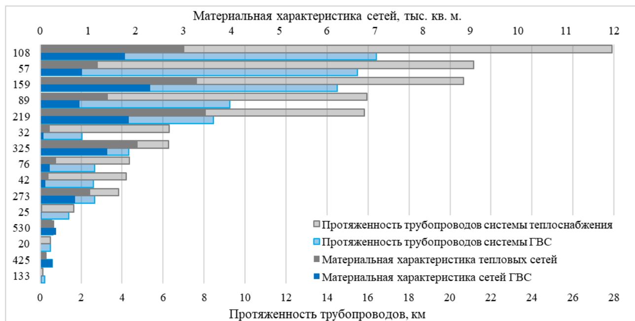
Рисунок 1. Структура сетей теплоснабжения и ГВС по диаметру трубопроводов
