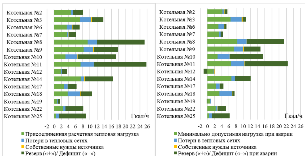
Рисунок 2. Баланс мощности источников в штатном и аварийном режимах
